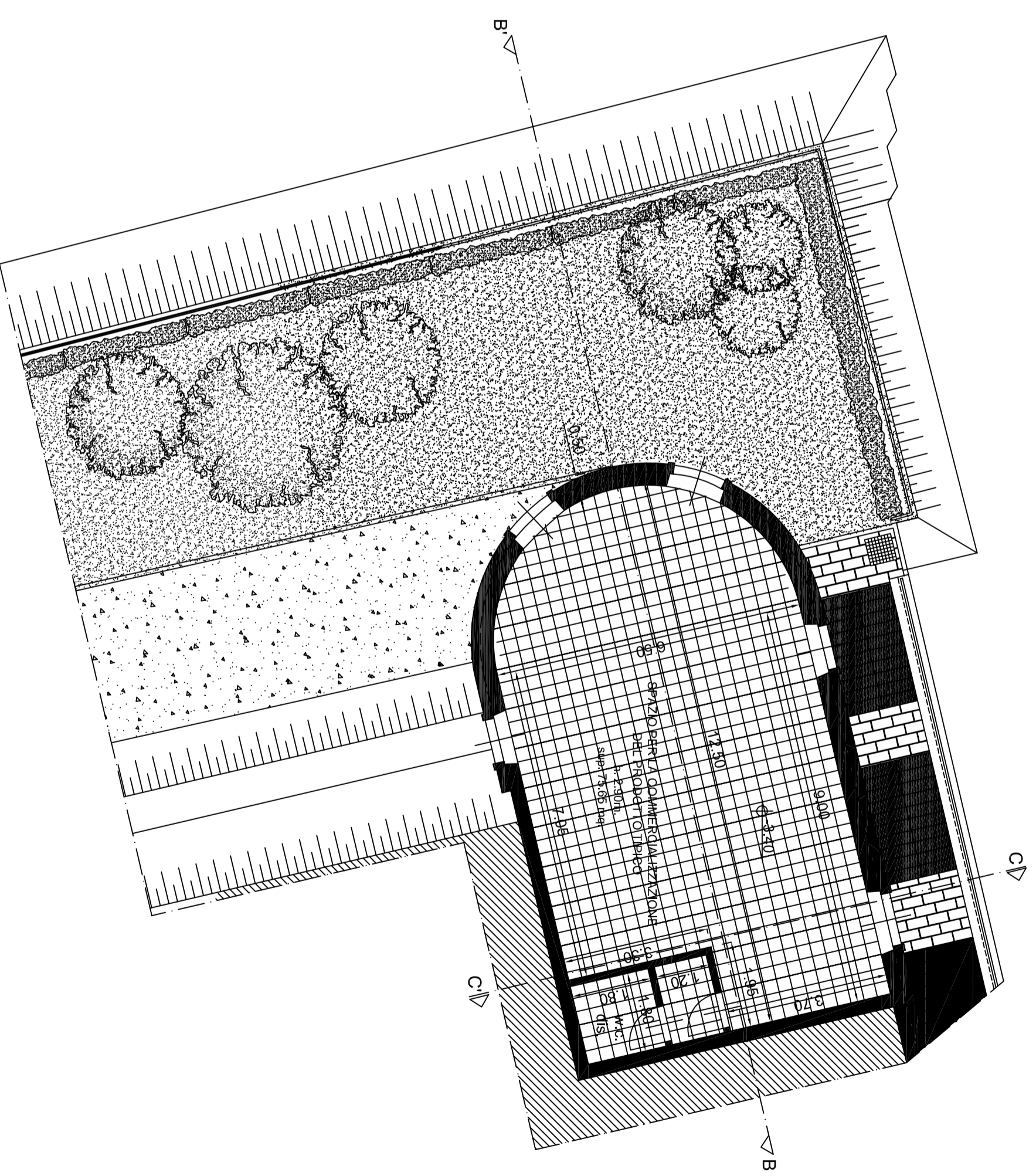
PIANTA A QUOTA -3.40
